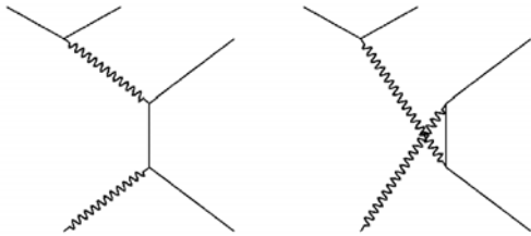
Bremsstrahlung Emission
